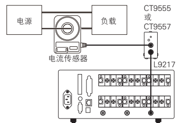
TYPE2 电流传感器连接示意图
