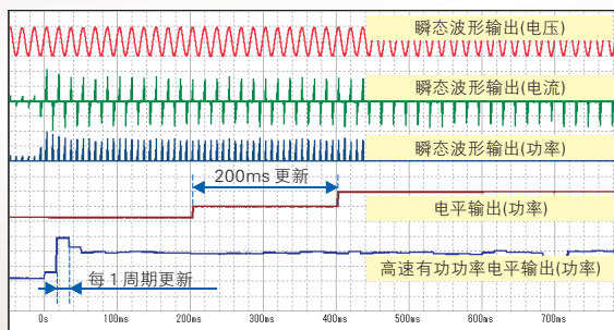
风扇马达启动时的D/A输出波形
